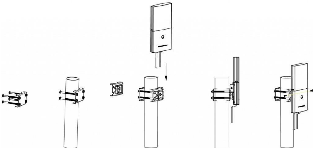
图 11 GWN7600 LR 纵杆安装
