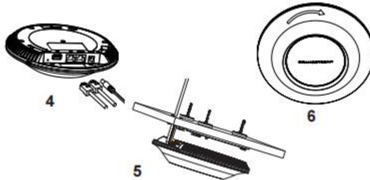
图 10 GWN76xx 顶式安装
