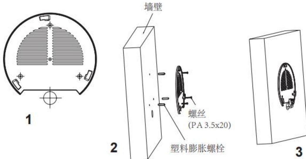
图 7 GWN7600 壁挂式安装
