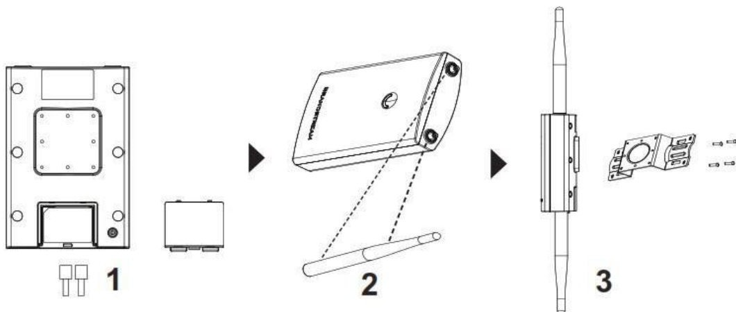
图 13 GWN7630LR/GWN7605LR/GWN7660LR /GWN7664LR 安装说明
