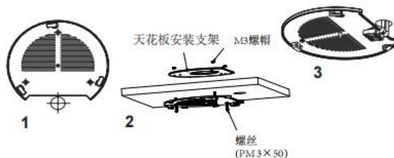
图 9 GWN76xx 顶式安装
